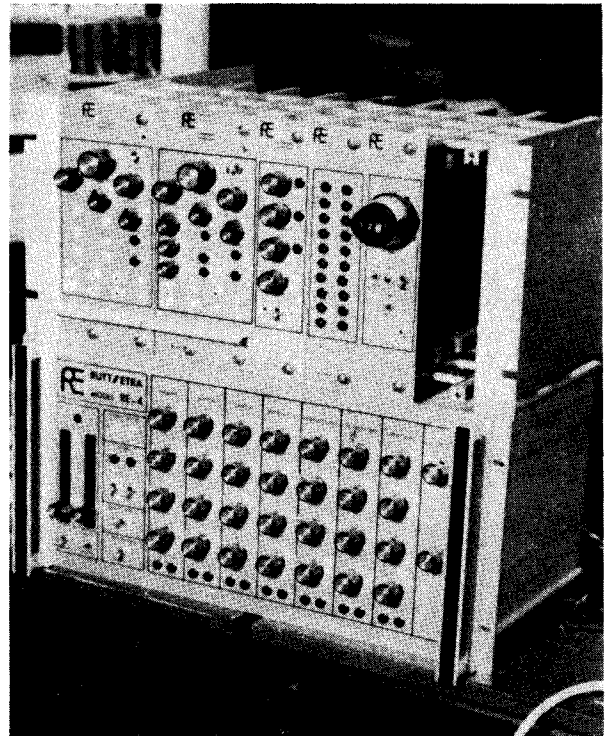
Synthétiseur Rutt/Etra
