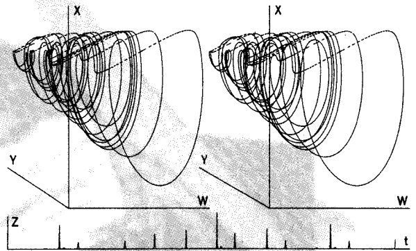
Otto E. Rössler, Hyperchaos-Gleichung
